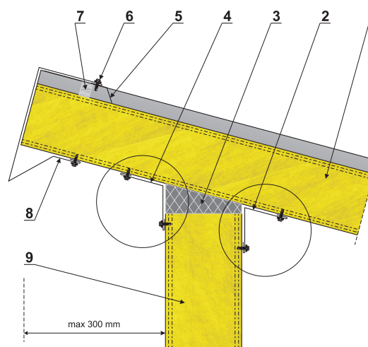
obróbka narożna OBR-PD-12
