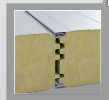
Zamek płyty ściennej
