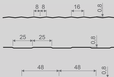
Rodzaje profilowania płyty ściennej
