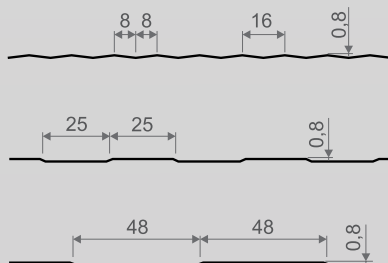
Rodzaje profilowania płyty ściennej akustycznej
