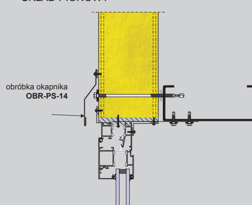
Obróbka okna - góra UKŁAD PIONOWY
