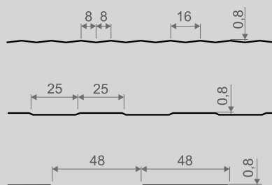
Rodzaje profilowania płyty ściennej EKO
