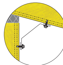
obróbka narożna OBR-PD-13
