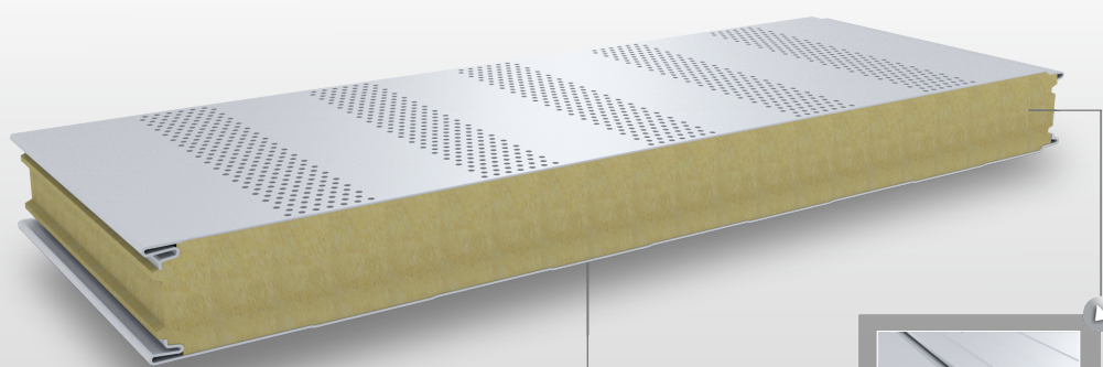
Płyta warstwowa ścienna akustyczna PWS-WA 100 mm
