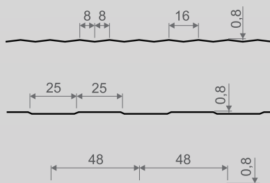
Rodzaje profilowania płyty dachowej
