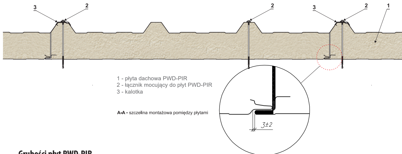
Rysunek 3 Płytę łączymy za pomocą trzech łączników na szerokości. Ważne jest zwrócenie uwagi na prawidłowe zamontowanie środkowego łącznika i odpowiednie uszczelnienie miejsca połączenia.
