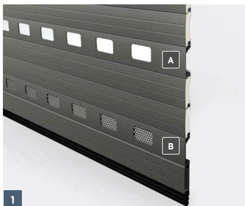
1 Kurtyna bramy – wykonana z profili aluminiowych o wysokości 100 mm i grubości 25 mm wypełnionych bezfreonową pianką poliuretanową. (A) – jednościankowy aluminiowy profil przeszklony, (B) – jednościankowy aluminiowy profil wentylowany.
