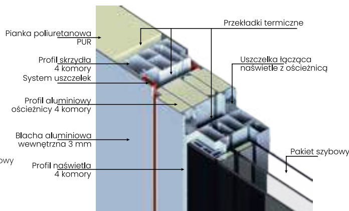
PROFIL OŚCIEŻNICY
