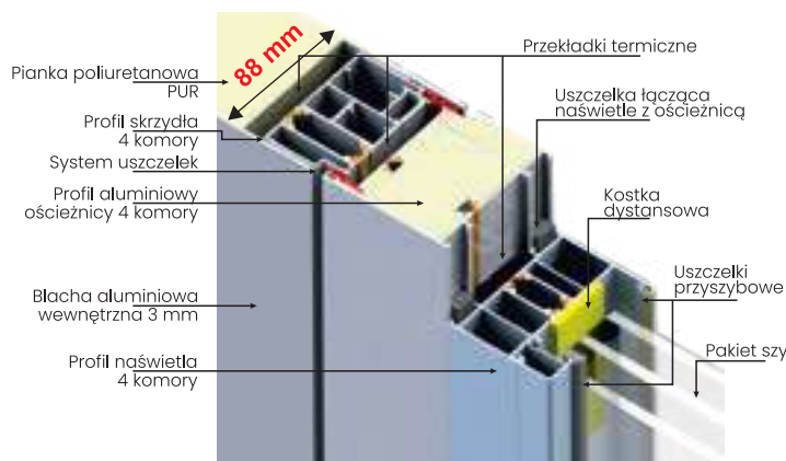
PROFIL OŚCIEŻNICY
