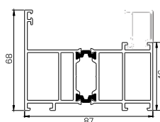
PROFIL NAŚWIETLA
