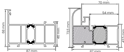
PROFIL NAŚWIETLA PROFIL OŚCIEŻNICY ALU/90
