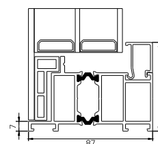
PROFIL NAŚWIETLA
