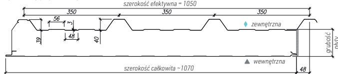
PIRTECH płyta warstwowa dachowa
