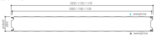
PIRTECH płyta warstwowa chłodnicza
