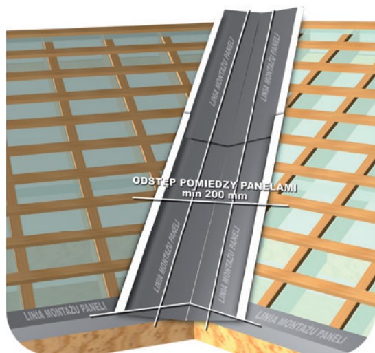
RYS. 18 Montaż rynny koszowej
