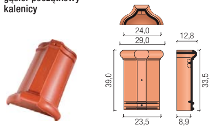
gąsior początkowy kalenicy
