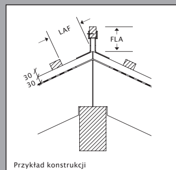
Przykład konstrukcji
