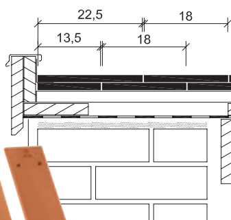
Szczyt z wiatrownicą, rynienką i karpiówkami 1 ¼ i ¾
