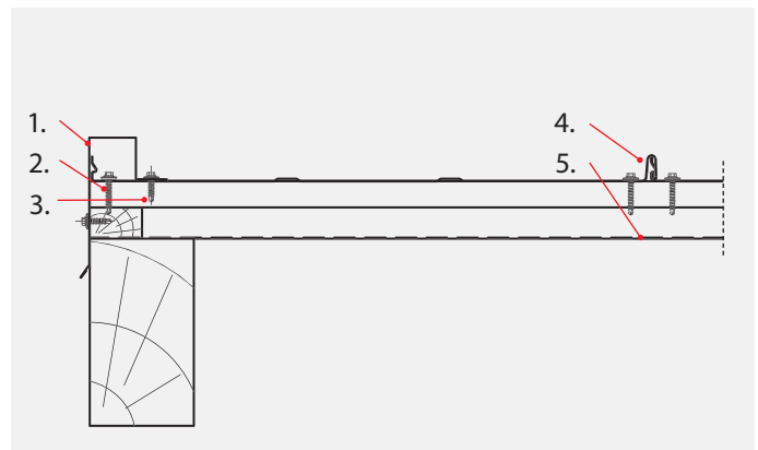
RYS. 44. ROZWIĄZANIE W SZCZYCIE DACHU
