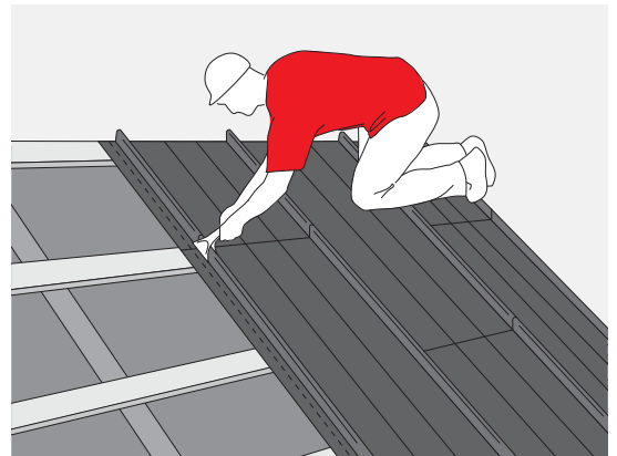
RYS. 30. ZACISKANIE ZAMKA PANELI W ZAKŁADACH
