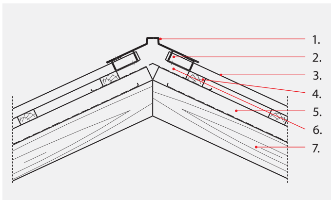
RYS. 43. PRZEKRÓJ DACHU W KALENICZY
